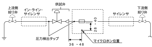
図1 ISA-RP59.1によるラボラトリ・テスト装置
