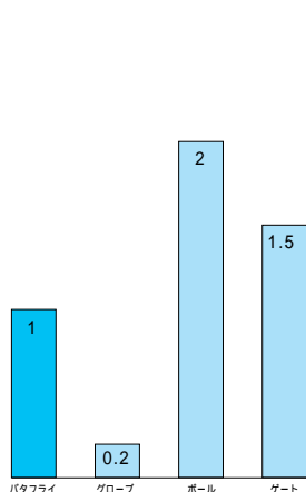
各バルブのCv値の対比 (バタフライバルブを1とする)
