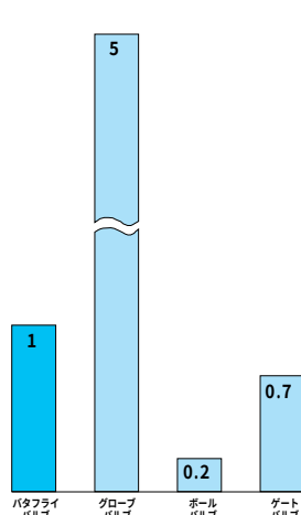
各バルブの圧力損失の対比 (バタフライバルブを1とする)
