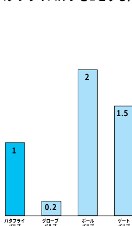
各バルブのCv値の対比 (バタフライバルブを1とする)
