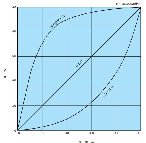
固有流量特性
